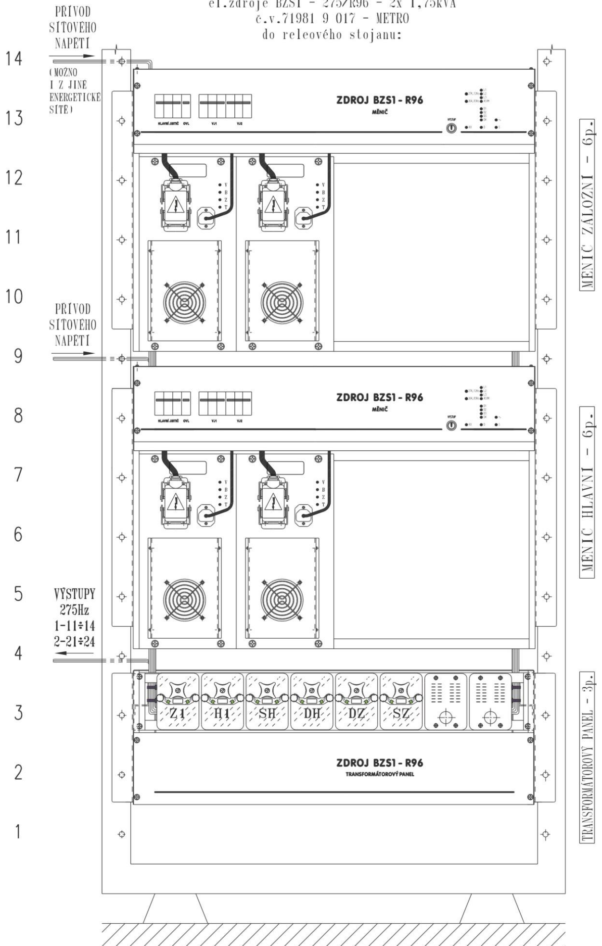
Příloha 3: Blokové schéma zdroje BZS1 - 275/R96
